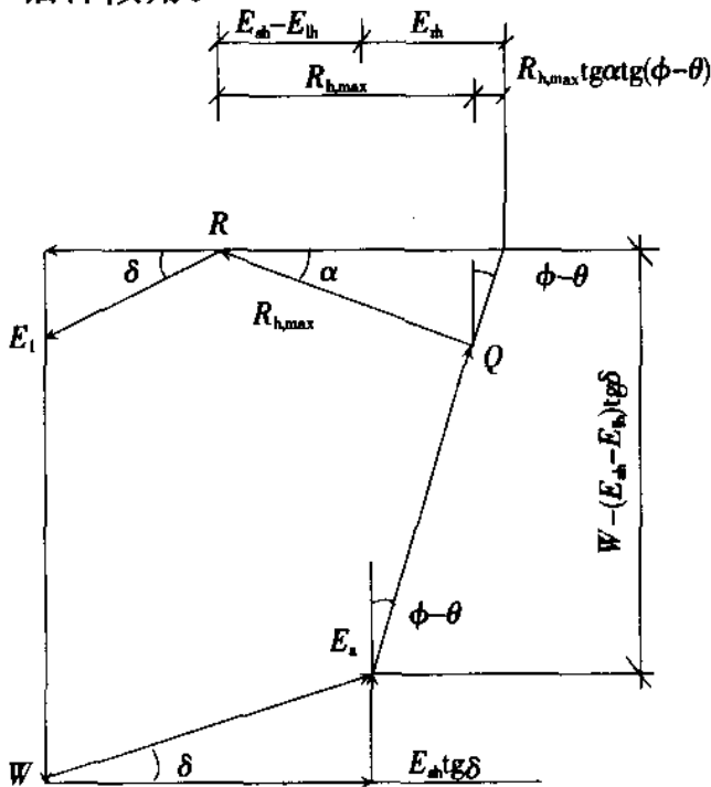
图 7 力多边形几何关系
