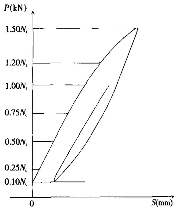
图 F 锚杆荷载-位移曲线
