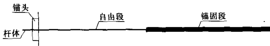
图 4.2.1 拉力型预应力锚杆结构原理
